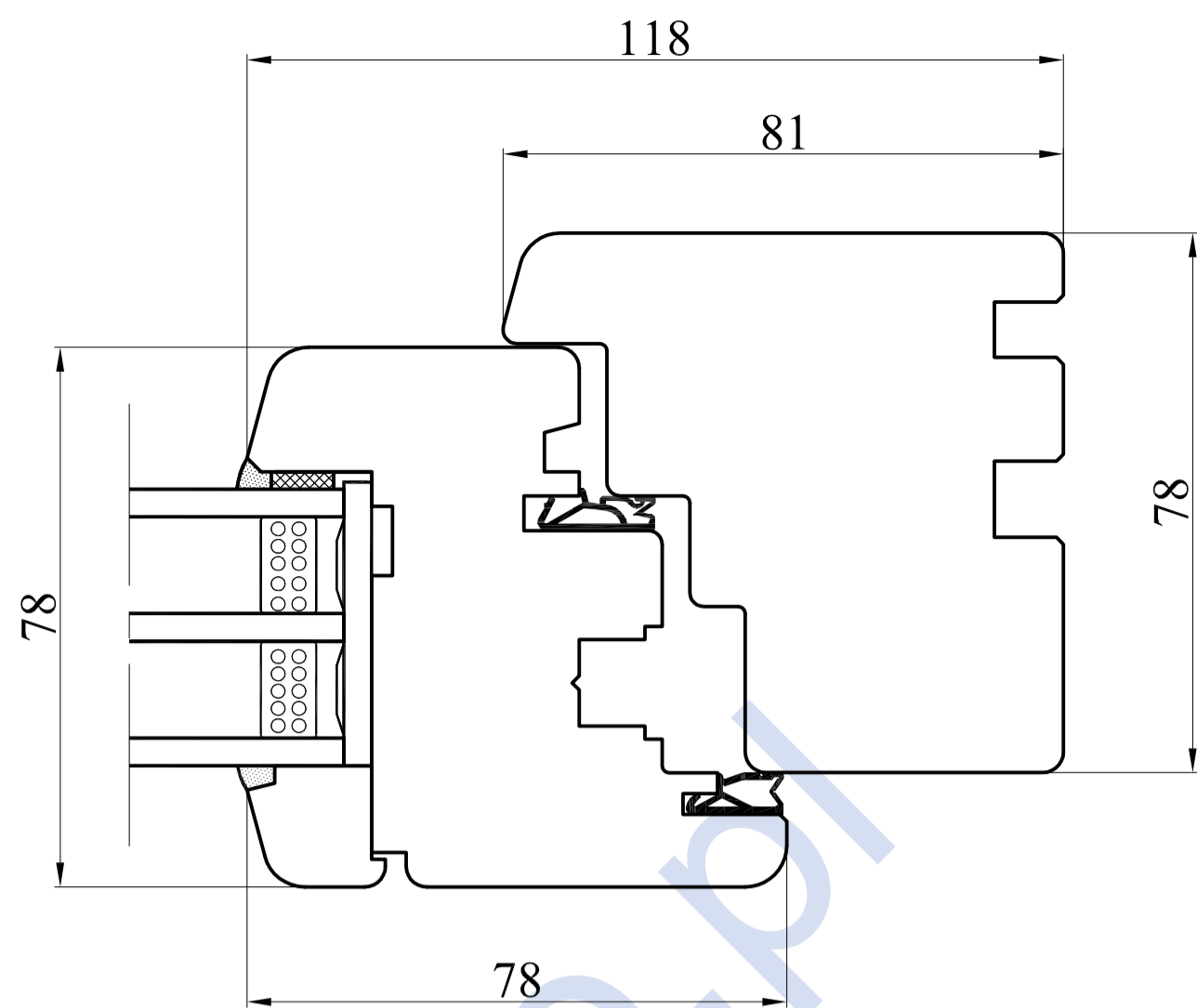
Przekrój B-B
